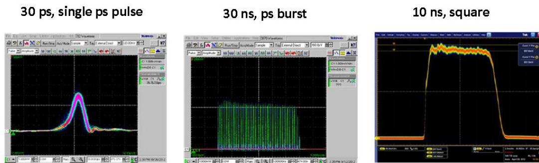
图 2、时域波形展示图例
