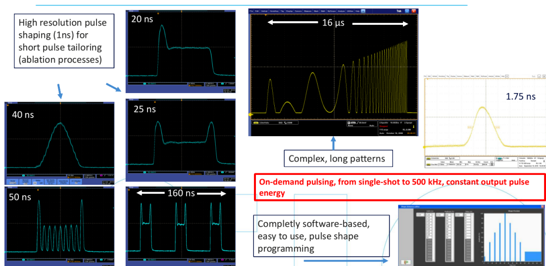
图 3、纳秒（ns）时域波形图实例
